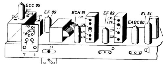
Chassis von hinten
