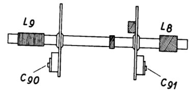
Ableichelemente der Ferritantenne
